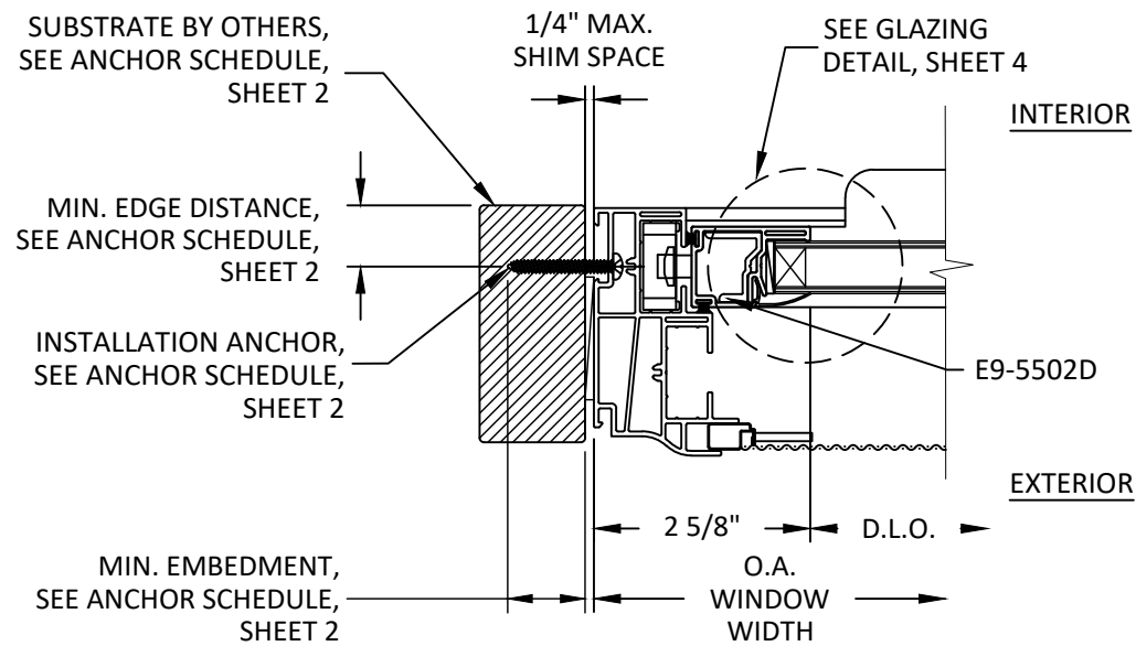
D 4 HORIZONTAL SECTION LOWER VENT JAMB
