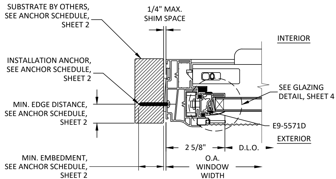
E 4 HORIZONTAL SECTION UPPER VENT JAMB
